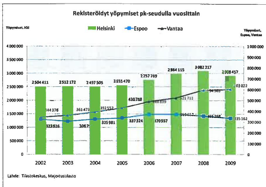
Kuva 1. Yöpymiset pääkaupunkiseudulla 2002-2009
